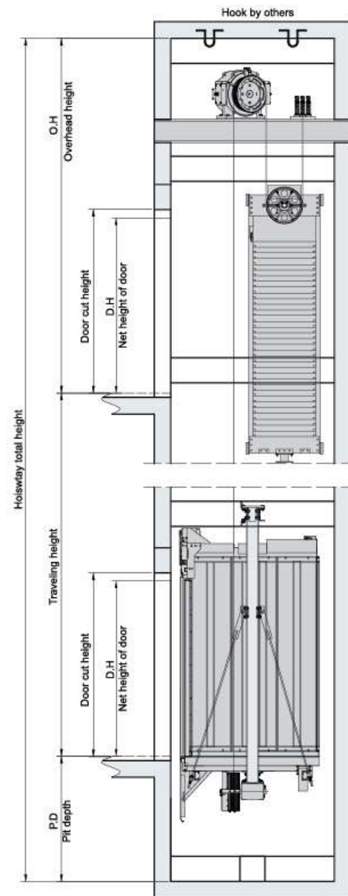
Hoistway elevation
