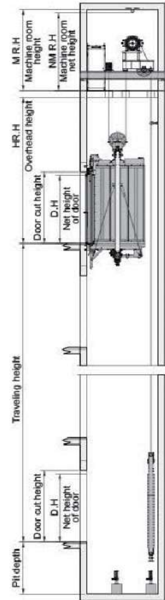
Hoistway elevation
